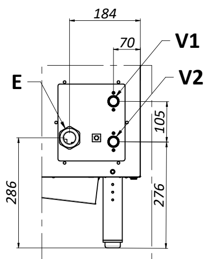
DETTAGLIO B
